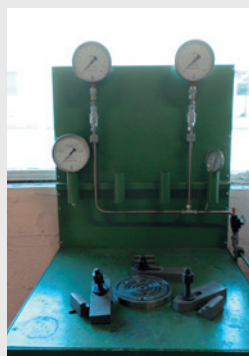
Banc de tarage de soupapes et tests de vannes
