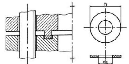
Joint de type "ED" pour brides à emboîtement double "ED" type gasket for tongue/groove face flanges
