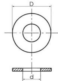
Joint de type "I" pour brides à face plate ou surélevée
